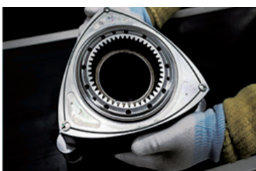
e-SKYACTIV R-EVのローター
